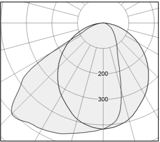
AREL asymmetrisk afskærmning for tavlebelysning
