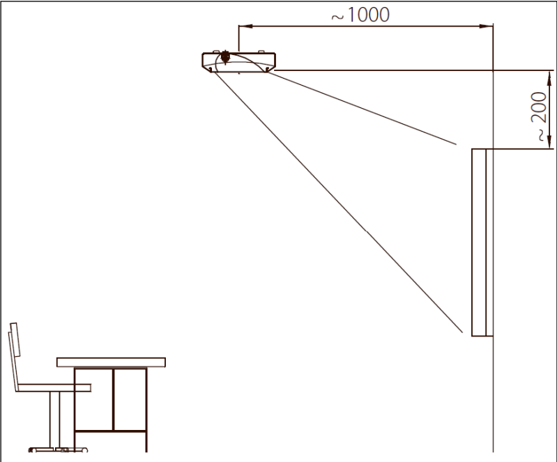
AREL asymmetrisk afskærmning for tavlebelysning. Illustration her viser fordeling af lys mod eksempelvis en tavle.
