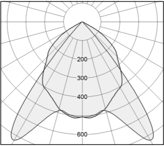
AREL med mat reflektor afskærmning (standard type)
