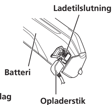
<BT-E8010/BT-E8014>
