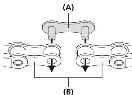
(A) Forbindelse af led med stifter
