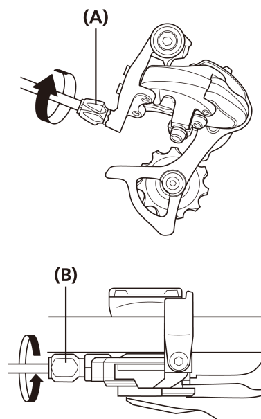
(A) Kabeljusteringsskrue (B) Justeringsbolt
