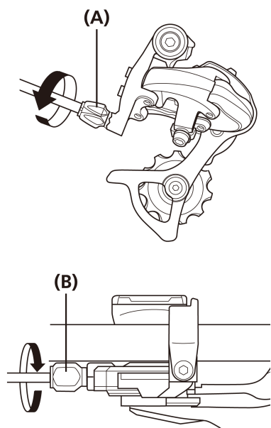
(A) Kabeljusteringsskrue (B) Justeringsbolt
