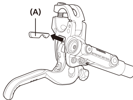
(A) Grebstopper
