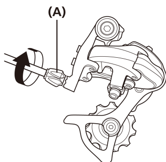
(A) Kabeljusteringsskrue
